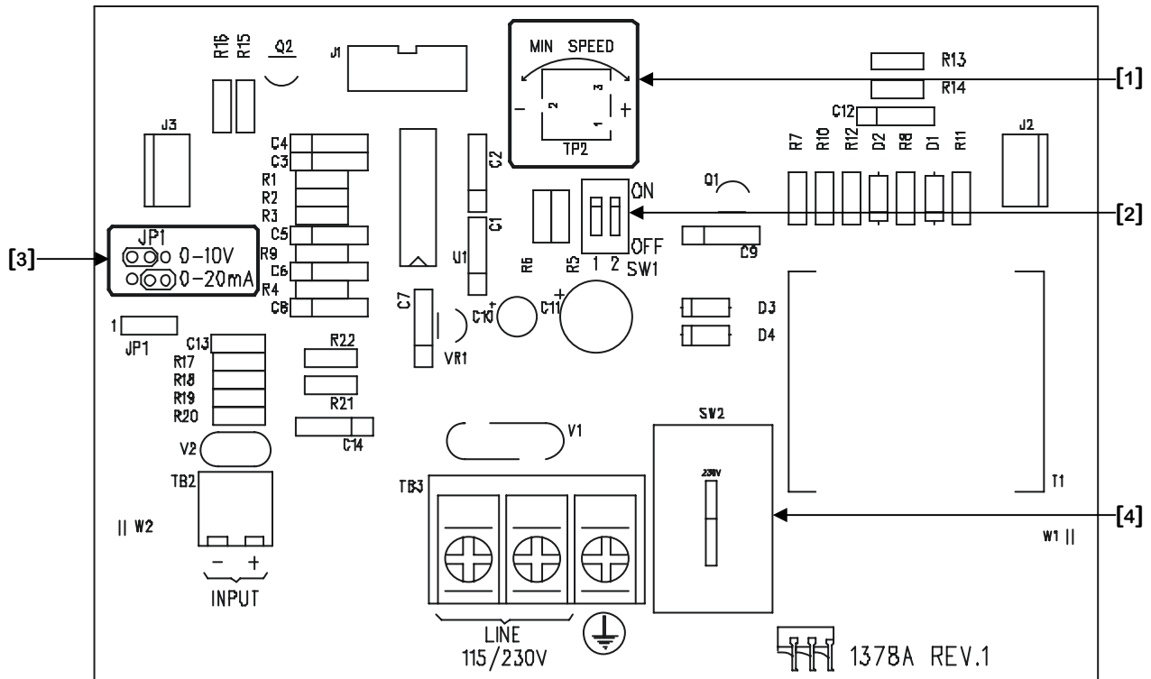
Figure 2: Localisation des composants sur la carte électronique
