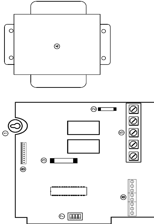
Fig.1 Vue d'ensemble de la carte électronique du SVIM-1/24LE
